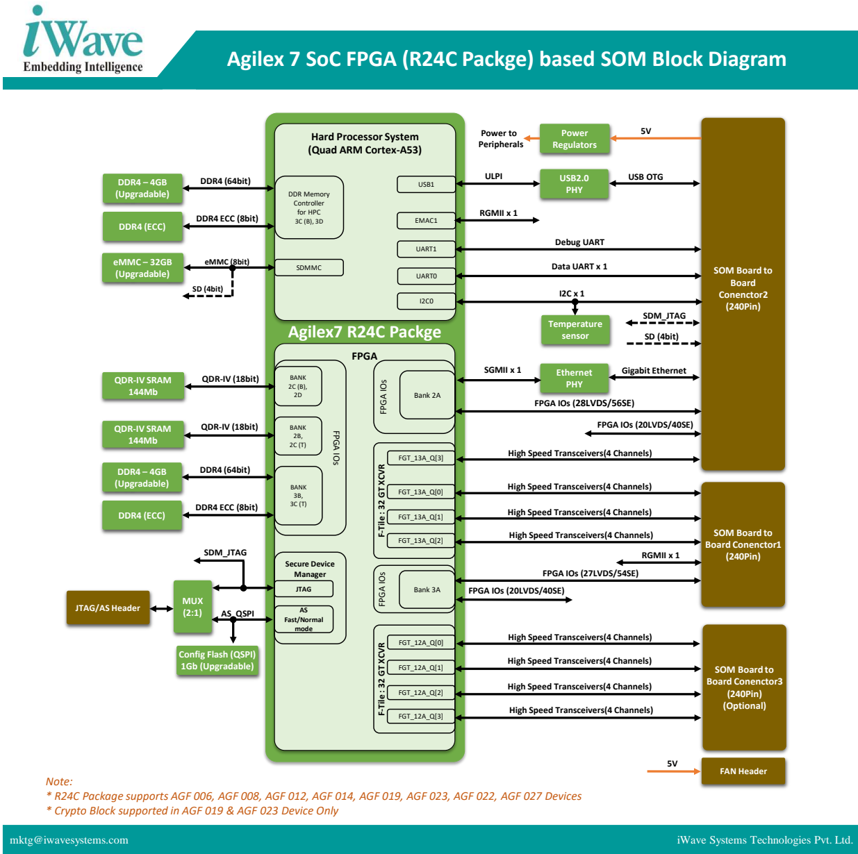
Figure 1: Intel Agilex 7 SoC FPGA SOM Block Diagram
